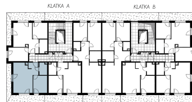
PLAN BUDYNKU
